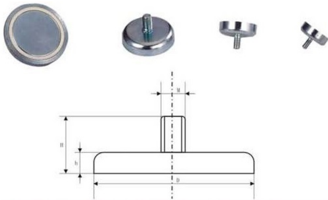
Uchwyt magnetyczny neodymowy z gwintem zewnętrznym C-20L 5mm Nikiel
